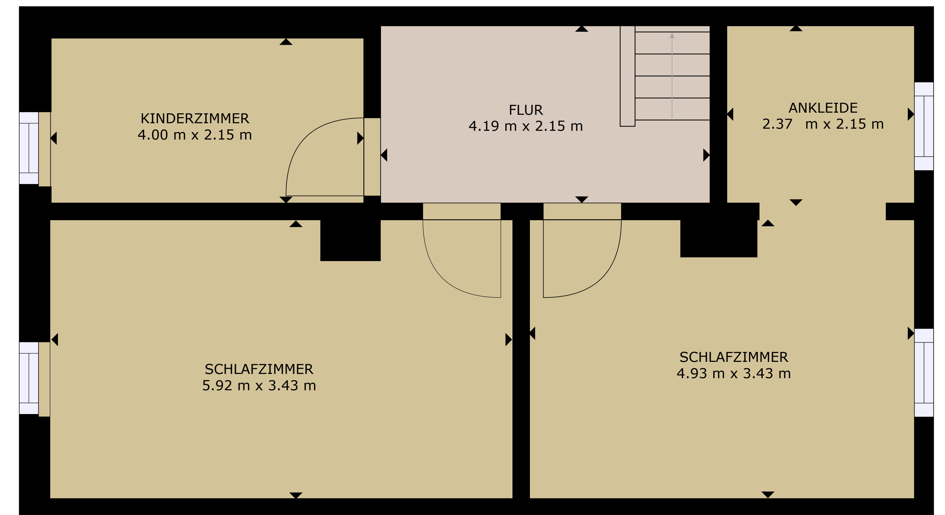
Dachgeschoss
